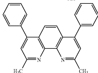
CBP
